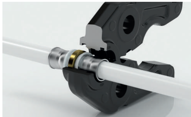
Matriz de prensagem TH
