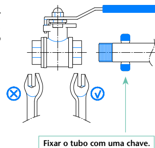
Fixar o tubo com uma chave.
