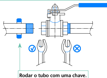
Rodar o tubo com uma chave.
