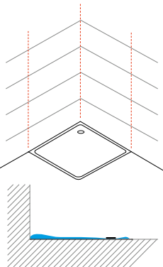
Cota zero . Zero quota . Quota zéro
