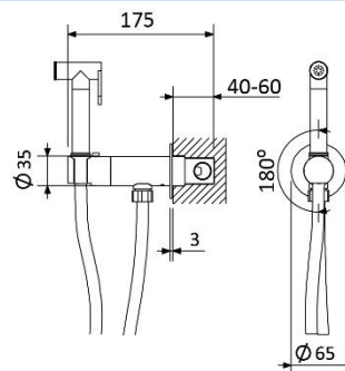
DESENHO DIMENSIONAL | DIMENSIONAL DRAWING
