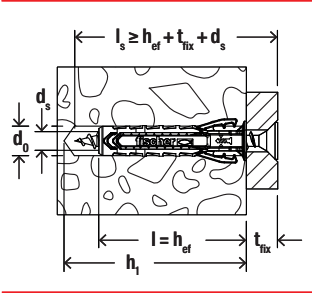
Bucha de expansão SX Plus Green
