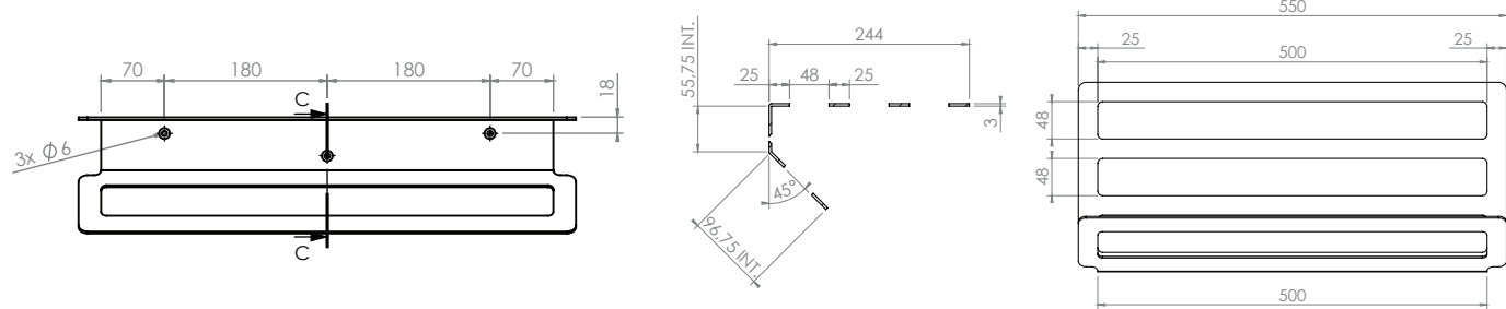
Toalheiro Duplo Alumínio Aluminium Double Towel Bar Ref. 1609
