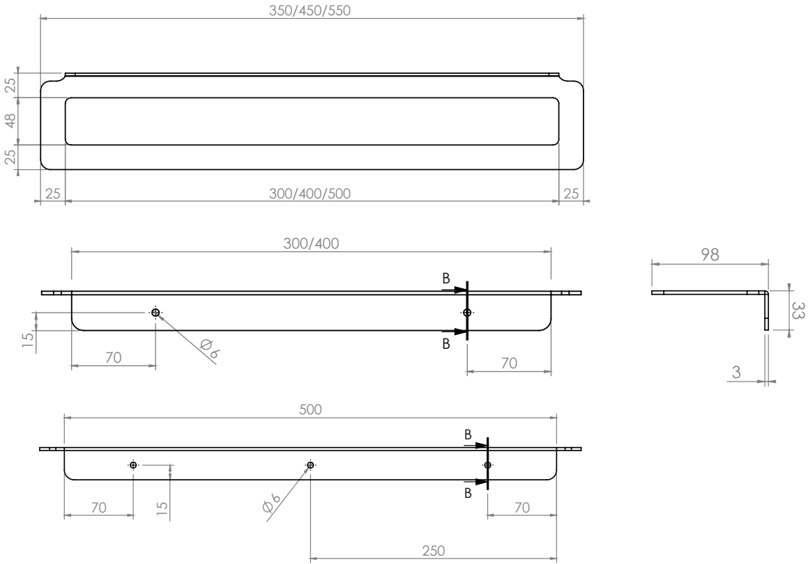
Toalheiro Duplo Alumínio Aluminium Double Towel Bar Ref. 1609
